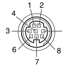
8-pol. Mini DIN-Buchse
