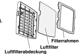
Luftfilterabdeckung
