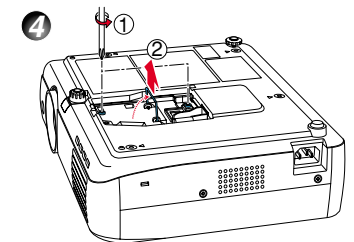
Lampenabdeckung
