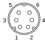
mini DIN 6-pin
